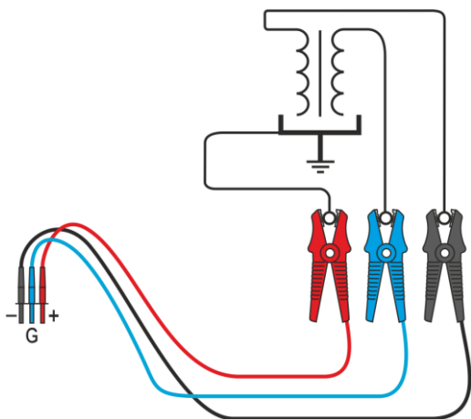
R iso- – przewód ekranowany
